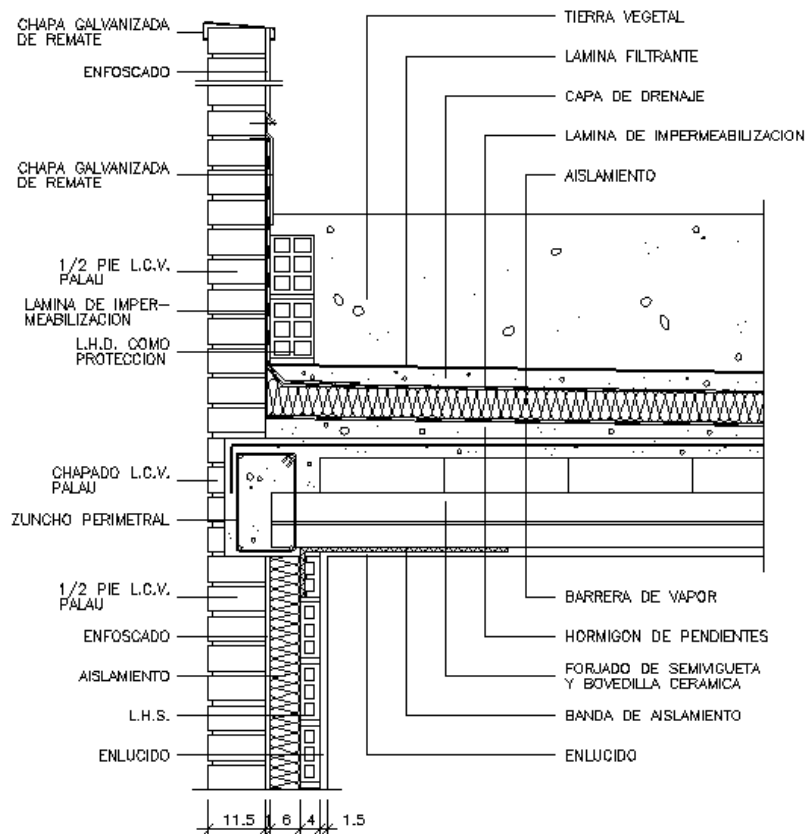
CUBIERTA PLANA AJARDINADA ESCALA 1:10 COTAS EN cm.
