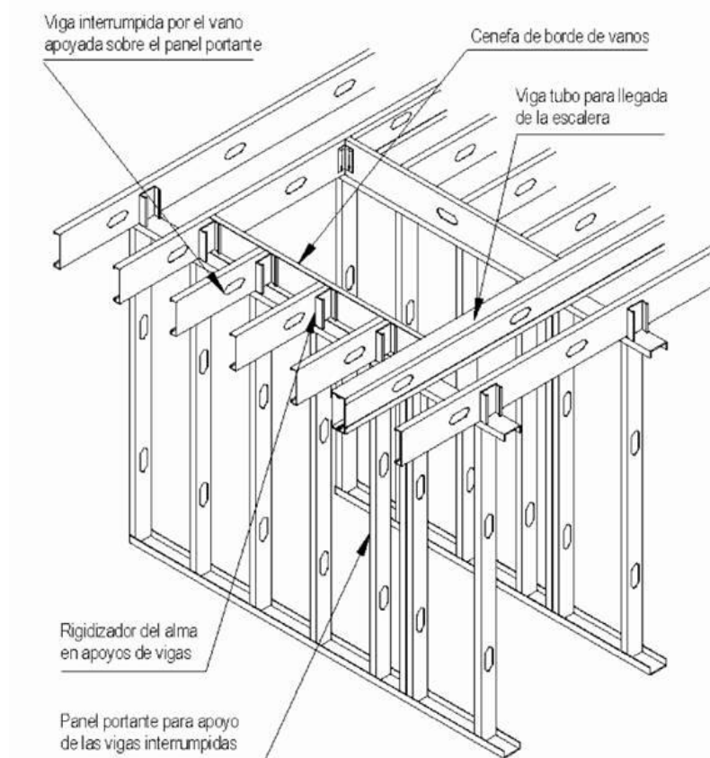
Figura 3.15. Viga tubo para llegada de escalera.
