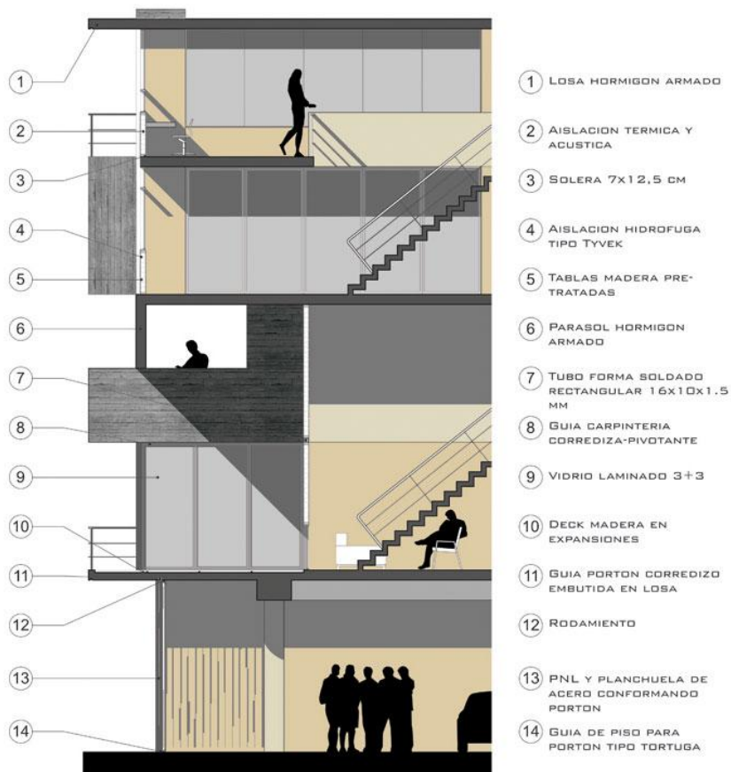
DETALLE ESC.: 1:25
