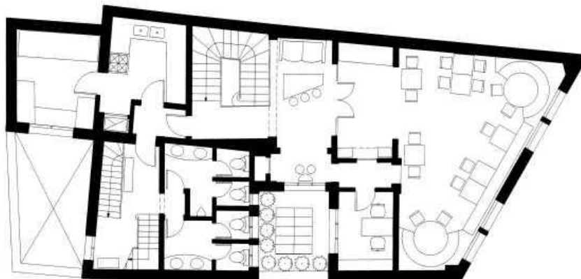
1º PISO
